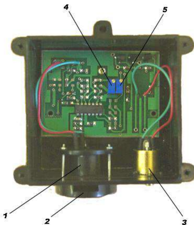
Рис.3. Датчик СИГМА-03.ДЭ со снятой крышкой. 1-Сенсор оксида углерода электрохимический; 2- фланец; 3 – вилка; 4 – потенциометр регулировки усиления; 5 – потенциометр регулировки начального тока.
